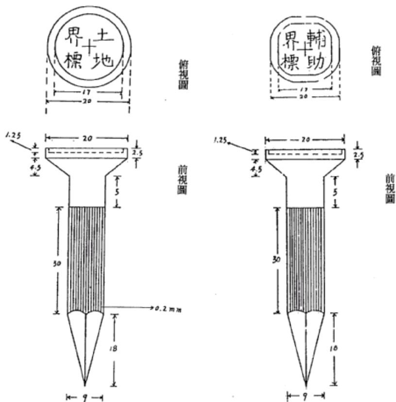
鋼釘界標（輔助界標）
